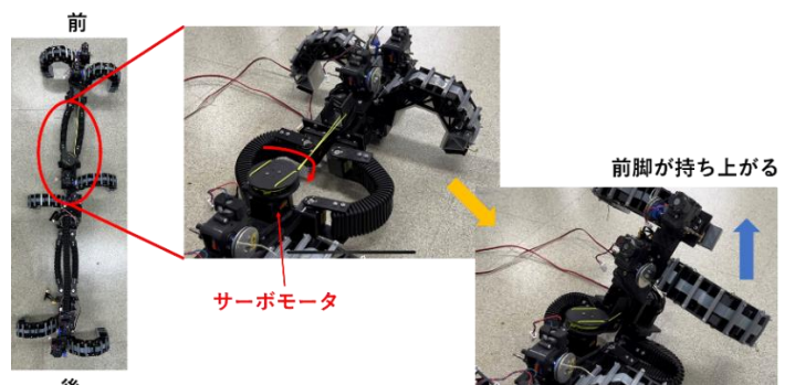
図 1 9 前脚持ち上げ機構
