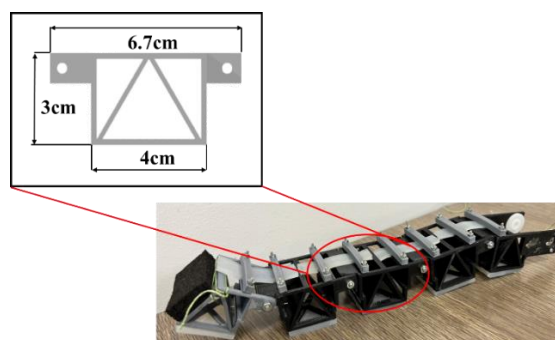
図5 作製した柔軟脚
