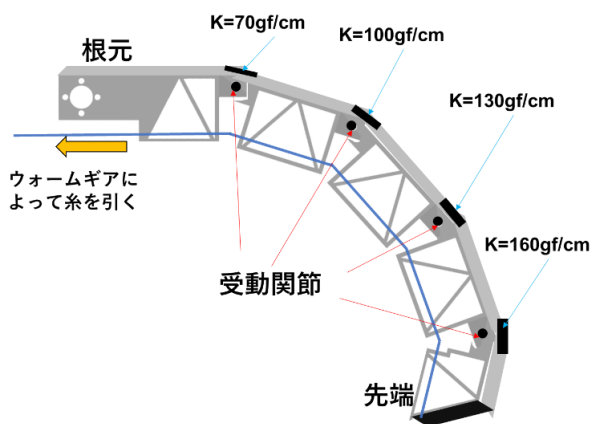
図6 柔軟脚の詳細
