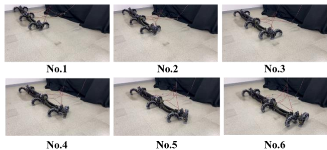
図 2 9 平面歩行実験
