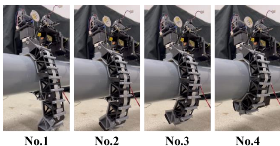
図9 実際に把持する様子
