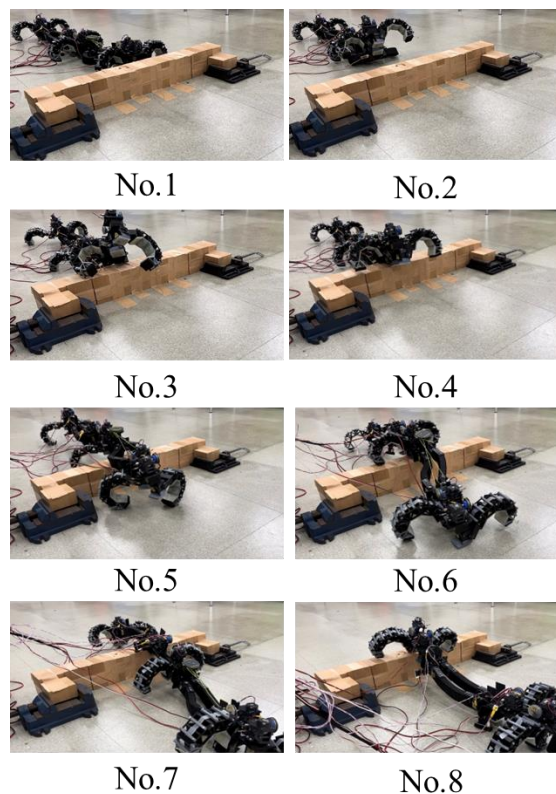
図 3 6 角柱走破実験
