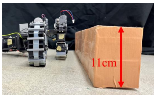
図 3 5 角柱走破実験環境
