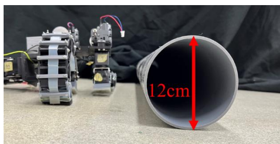
図 3 3 パイプ走破実験環境
