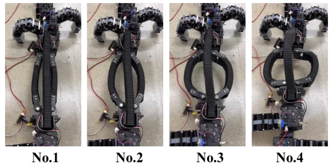
図 1 7 後胴体が縮む様子
