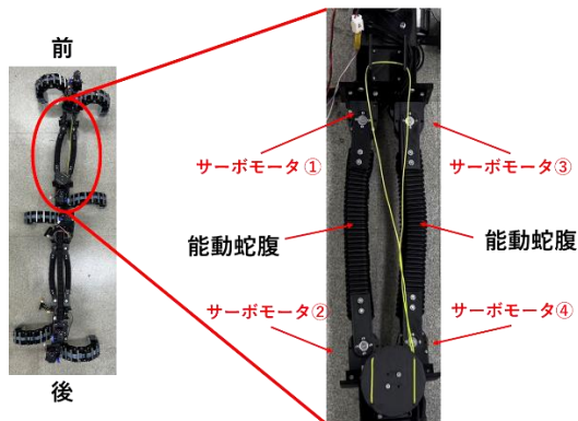
図 1 4 前胴体の機構
