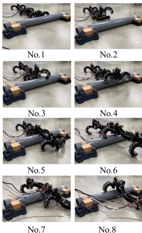
図 3 4 パイプ走破実験
