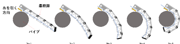
図7 パイプを把持する様子
