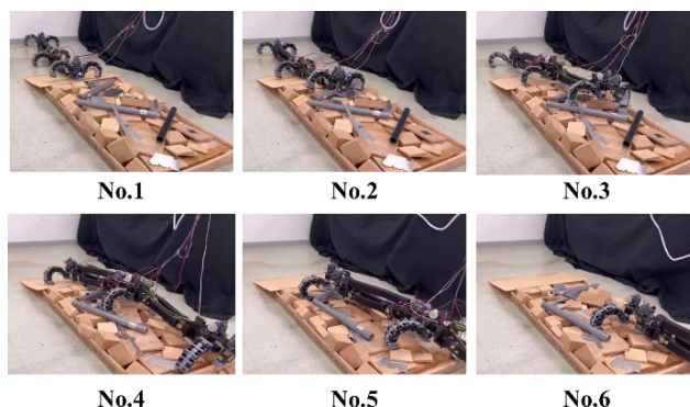
図 3 0 不整地歩行実験
