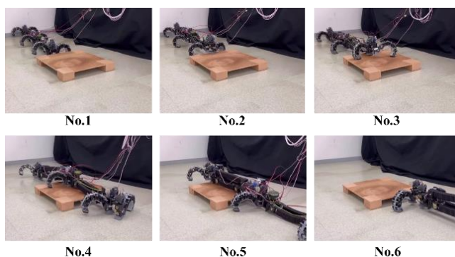
図 3 2 段差歩行実験
