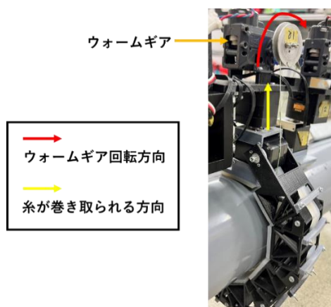
図8 ウォームギアの動き
