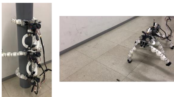
図2 従来機体 (TAOYAKA-V)
