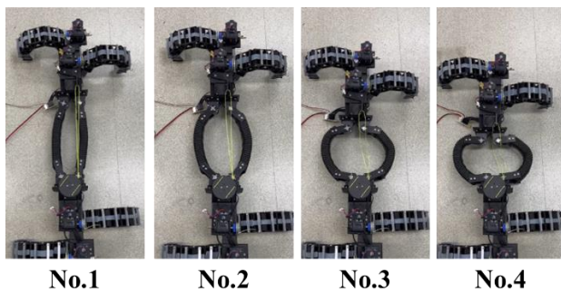
図 1 5 前胴体が縮む様子
