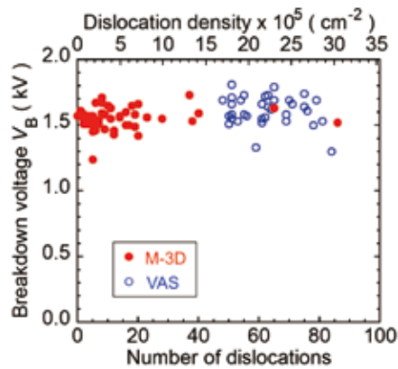
図5 逆方向耐圧のダイオード内転位数依存
