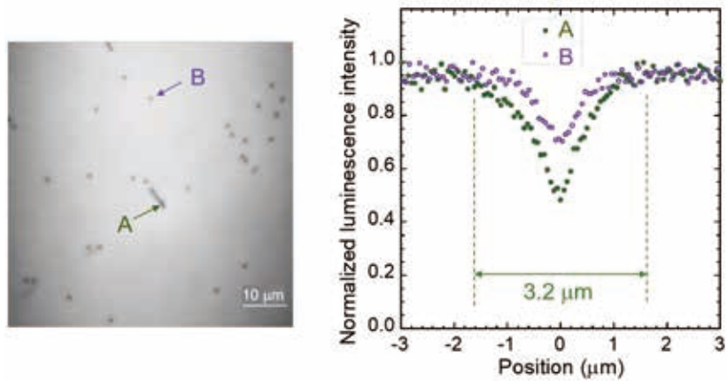
図4 2光子励起フォトルミネッセンスマッピング像と典型的な暗点の発光強度分布
