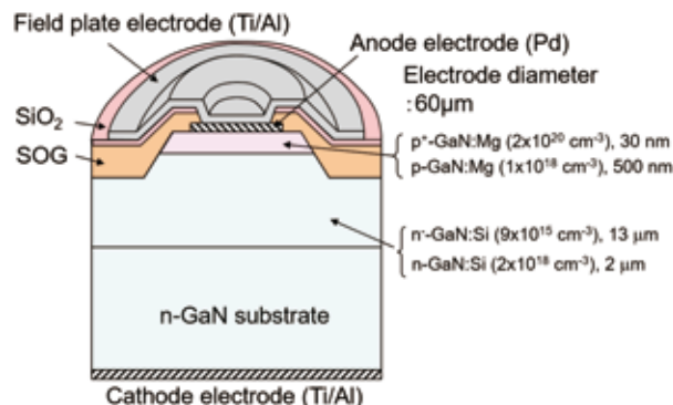
図1 GaN p-nダイオードの構造図
