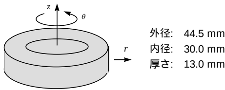
図3 フェライトトロイダルコア
