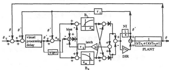
Fig. 2 シミュレーションモデル
