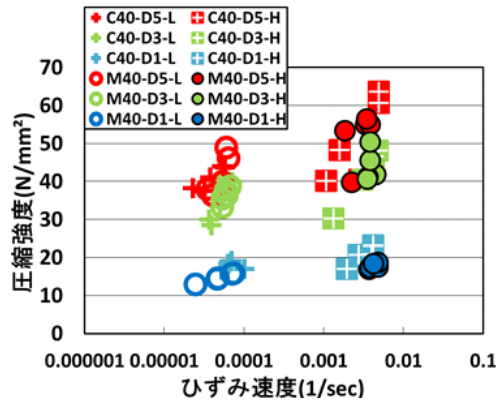
図 - 5 ひずみ速度 圧縮強度(弱材齢)
