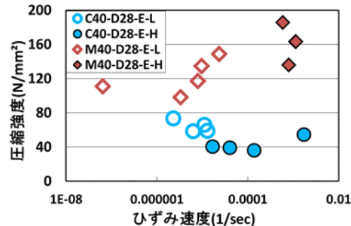
図 - 6 ひずみ速度 圧縮強度（凍結）
