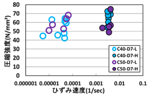
図 - 4 ひずみ速度 圧縮強度（標準）
