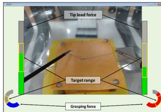
図4 提示システム
