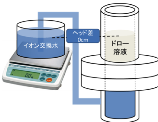
図1 吸水実験装置の概要
