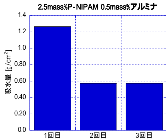
図2 PNIPAM+アルミナスラリーの吸水実験結果
