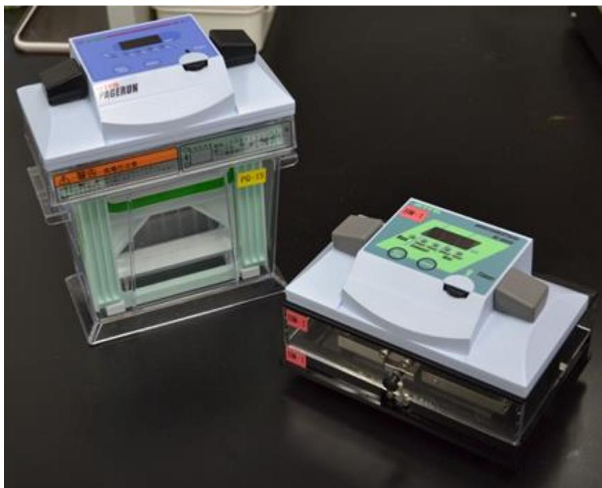
図3 ポリアクリルアミド電気泳動槽 PageRun (左) セミドライブロッターpowered BLOT mini (右)
