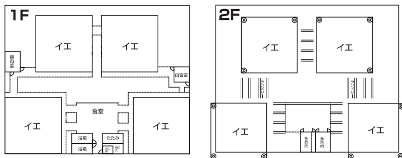
図3 寮全体の設計図案
