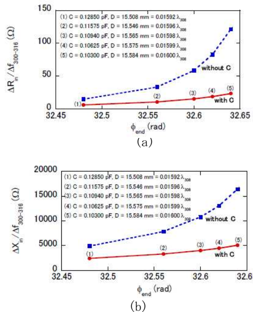
図8 入力インピーダンスの変化量 (a) 抵抗 R_{in} の変化量 (b) リアクタンス X_{in} の変化量
