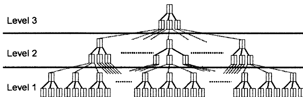
図 1: 部分木分散
