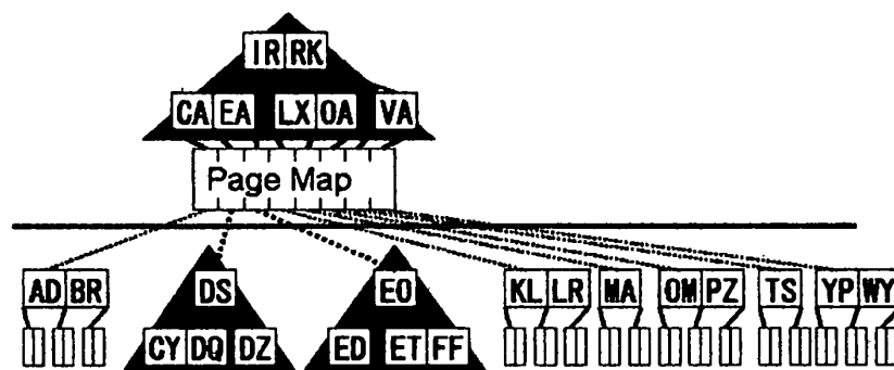
図 3: 部分木スプリット後
