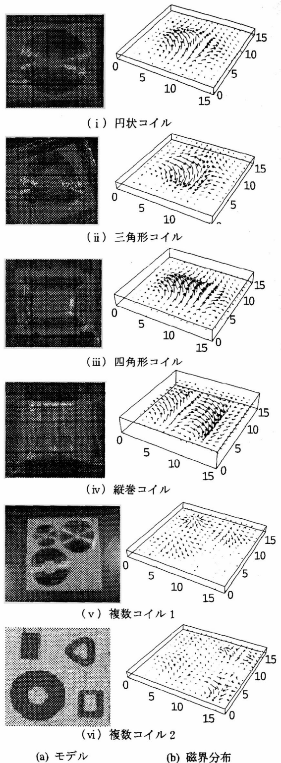
図8. 供試モデルと磁界分布の測定結果
