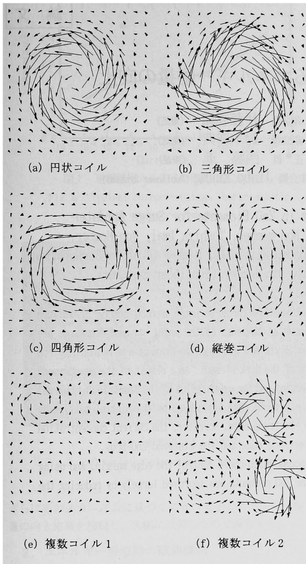
図9. 電流ベクトル分布 Fig. 9 Current vector distribution.
