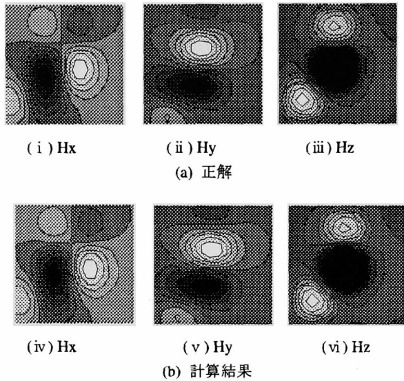
図7. 磁界分布
