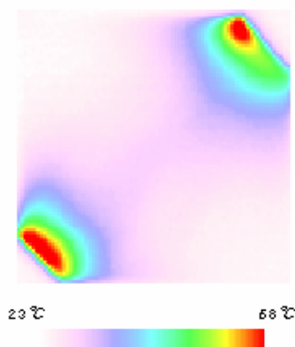
図 5.4 導電性繊維の絶対温度分布
