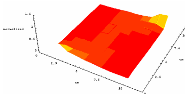
図 3.5 導電性繊維の x 軸方向の電位差分布
