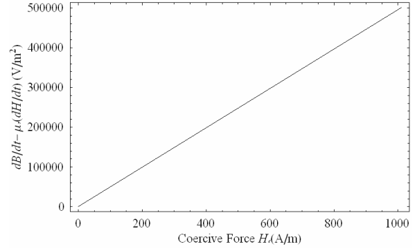
Fig. 3 Hysteresis Parameter s (TDK H5A).
