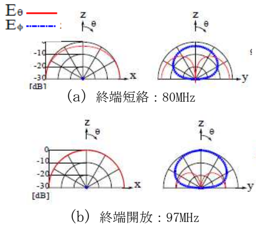
図6 放射パターン.
